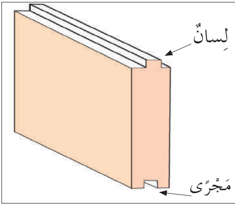
الشَّكْلُ (١٣-٣): وَضَلَّةٌ مَجْرَى وَلِسَانٌ.
